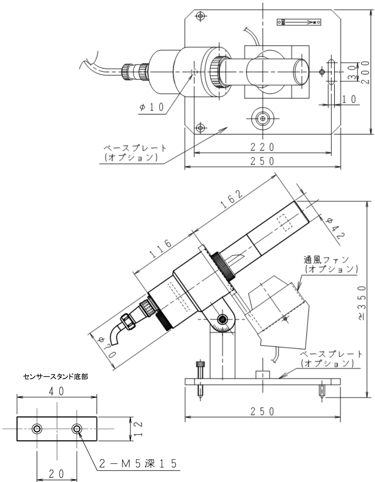
図 3-5. MS-093 寸法図
